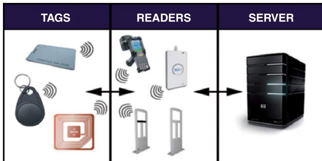
Tipica architettura RFID e rispettivi componenti
